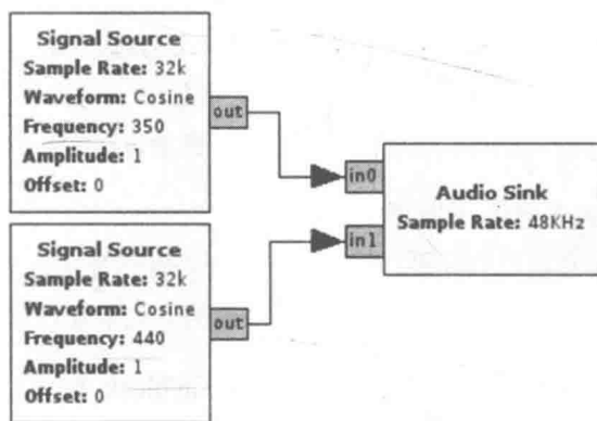
图9-18 产生拨号音的流图
