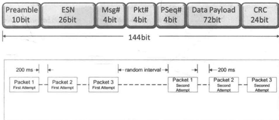
图8-33 数据包格式
