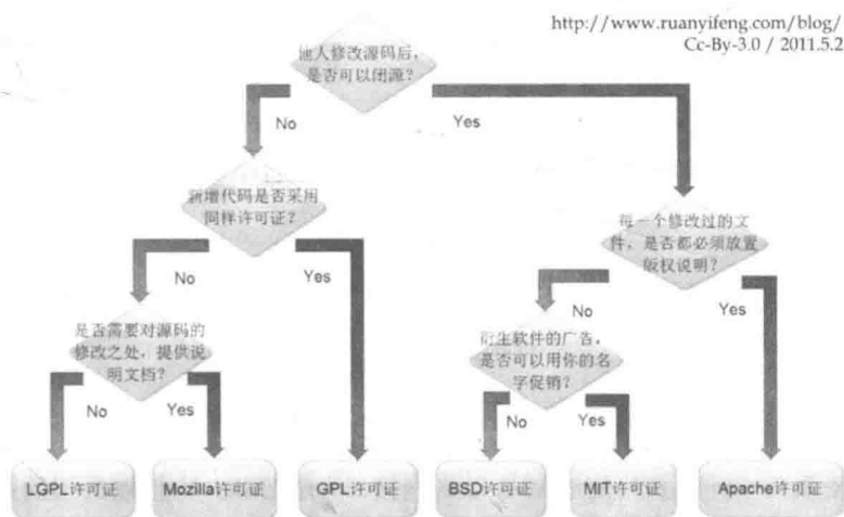
图9-2 几种开源软件许可的差别
