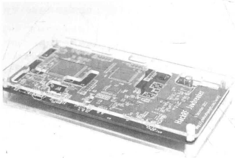
图9-10 HackRF的外观
