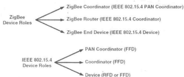
图6-3 ZigBee及IEEE 802.15.4中的设备角色 3
