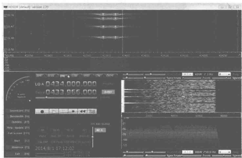
图 3-12 某奔驰车钥匙信号频谱图
