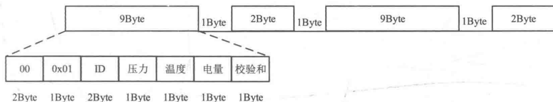
图3-30 胎压数据包格式
