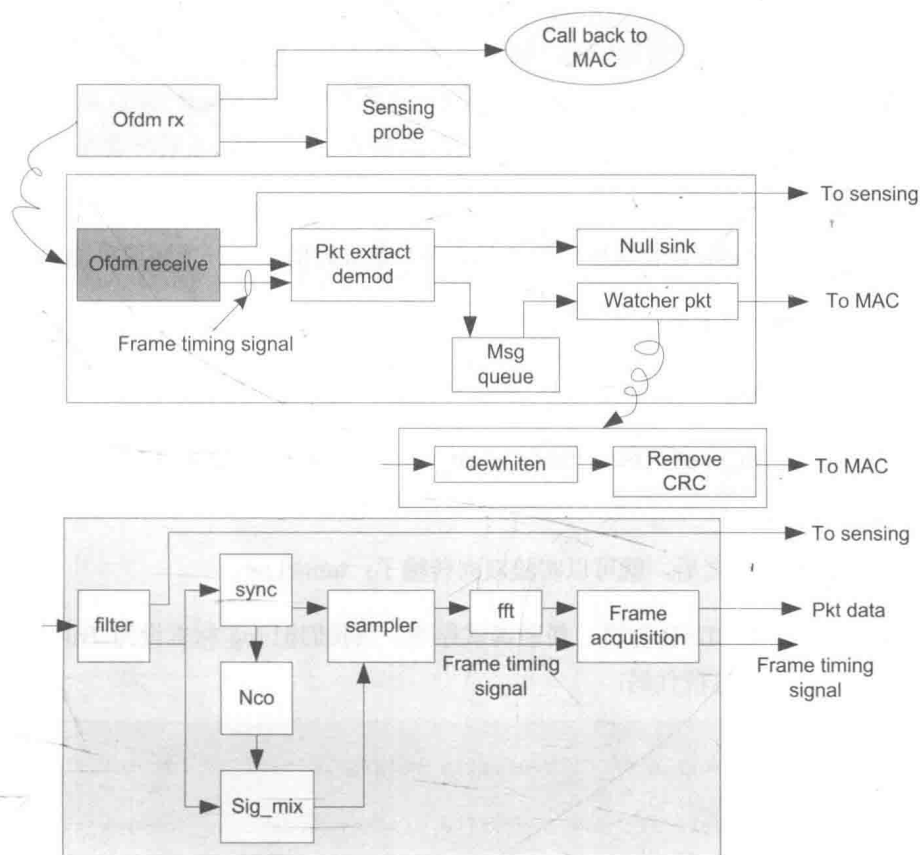
图9-24 OFDM Tunnel接收机框图
