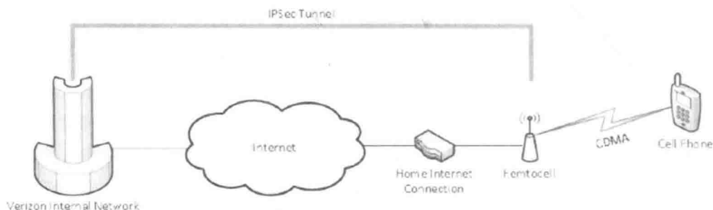
图7-23 三星家庭基站接入网络方式
