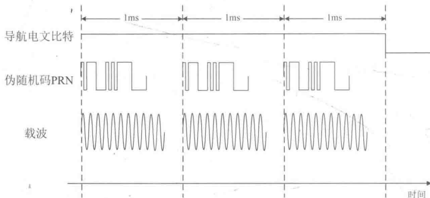
图8-9 GPS信号的基本构成示意图
