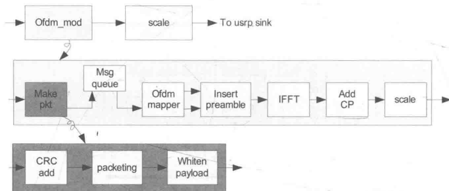
图9-23 OFDM Tunnel发射机框图
