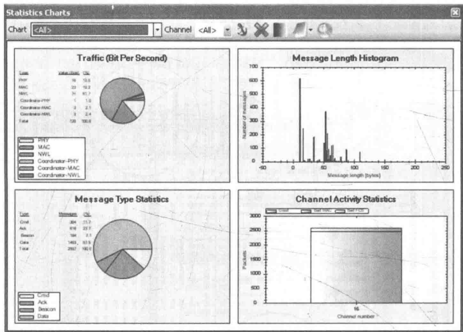
图6-18 Perytons Protocol Analyzer 8
