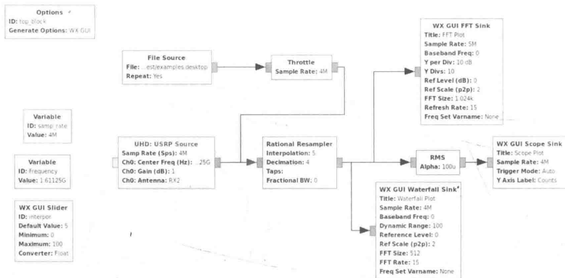
图8-30 上行链路信号捕获流图
