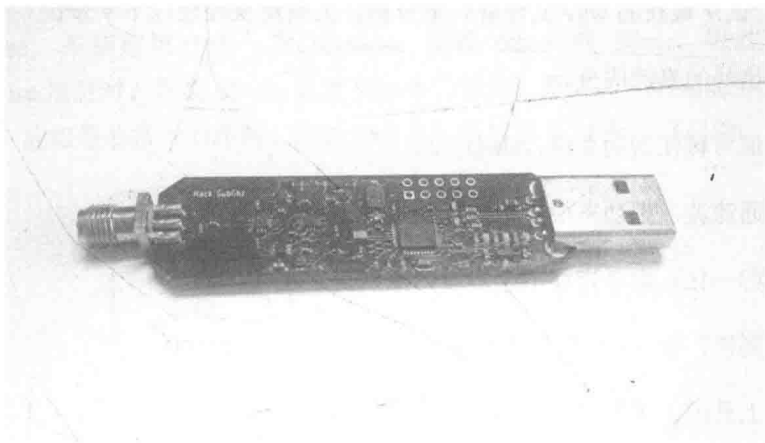
图3-22 Unicorn Team RF收发分析器
