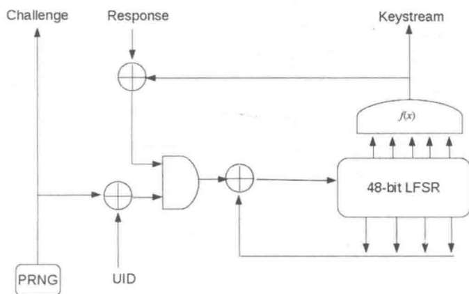
图2-3 Mifare Classic加密算法逻辑电路原理图
