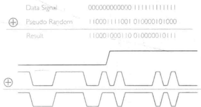
图8-24 PN码编码过程
