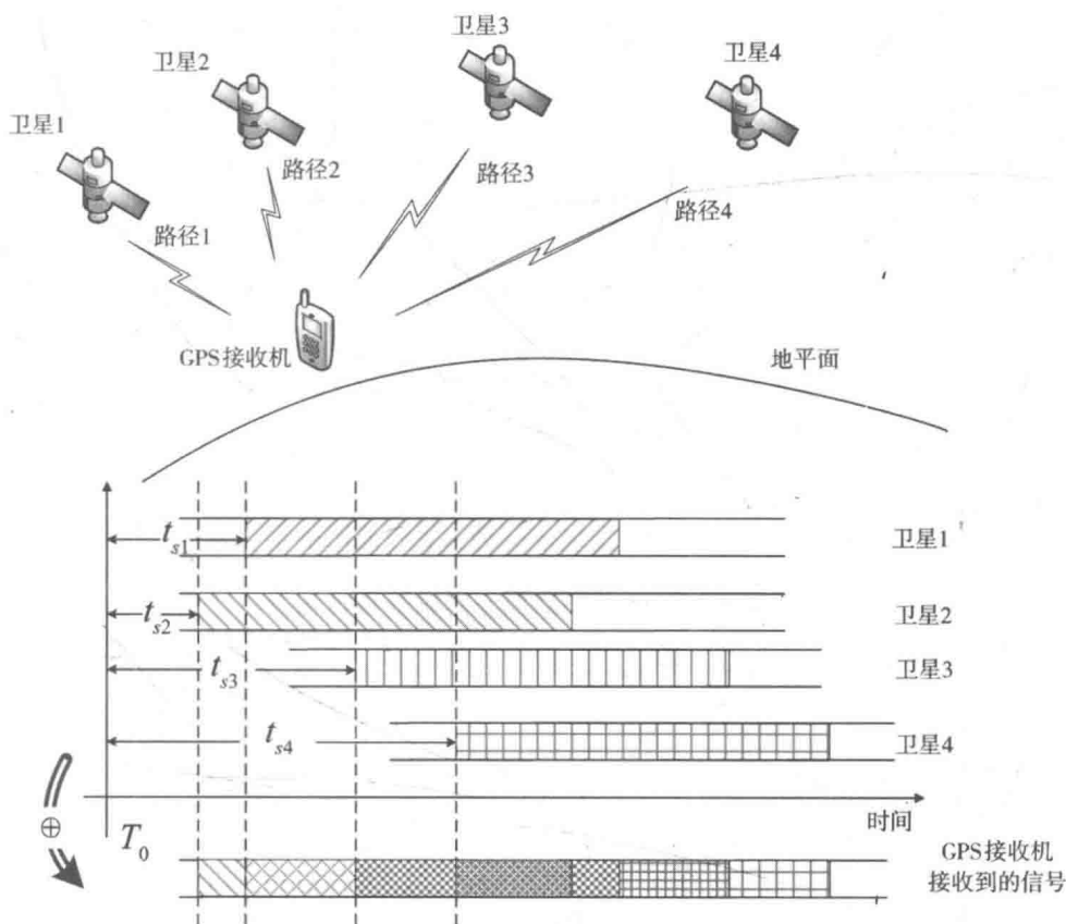
图8-8 GPS定位原理示意图
