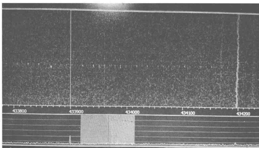
图3-28 传感器发射的信号
