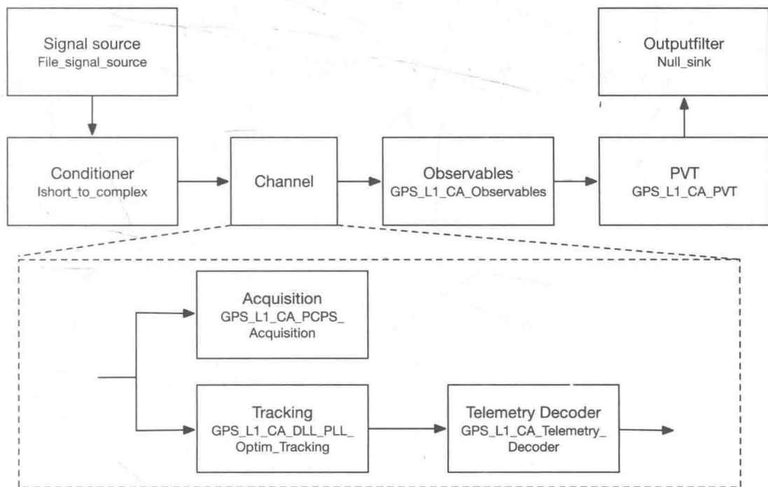
图8-11 GNSS软件无线电接收机模块连接框图
