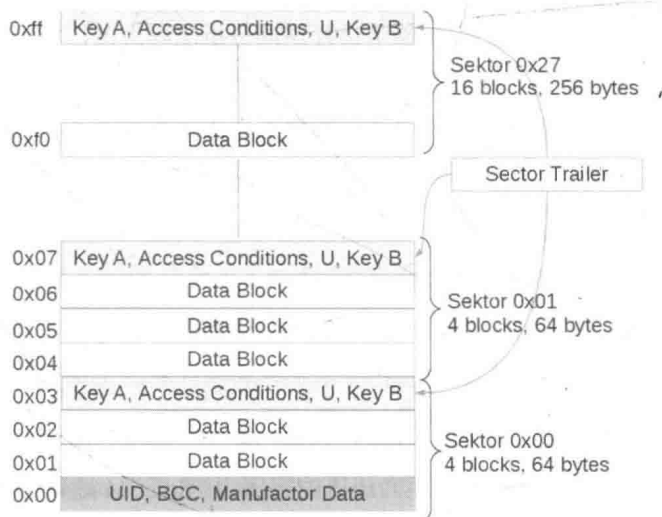
图2-1 4K Mifare Classic卡的扇区排列情况
