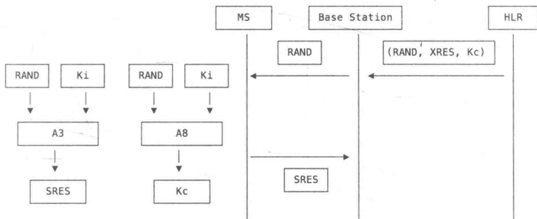
图7-1 A3/A8算法的实际使用流程图
