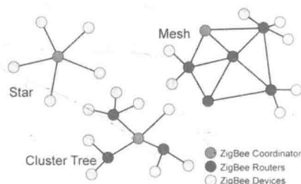
图6-4 ZigBee网络拓扑图 4
