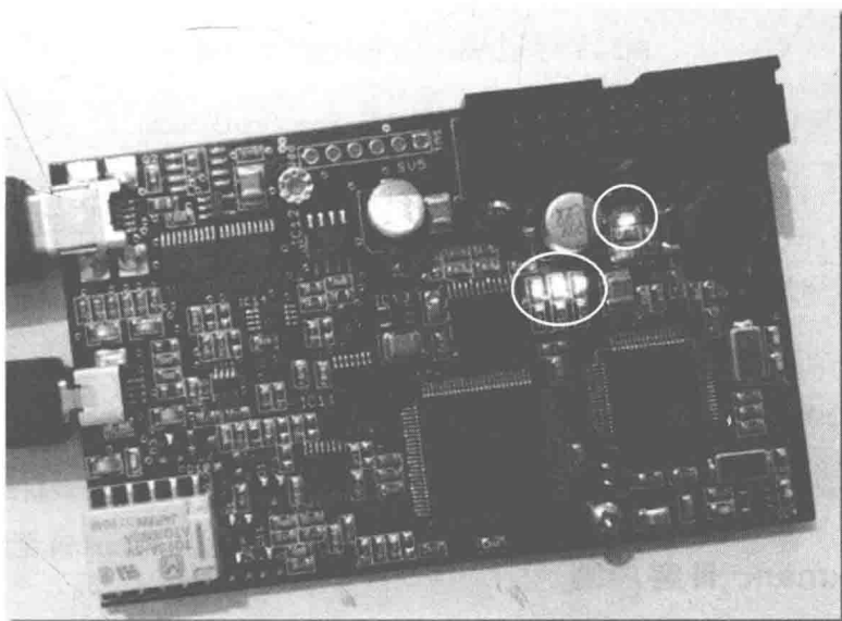
图2-13 Proxmark III板上的4个指示灯全部亮起
