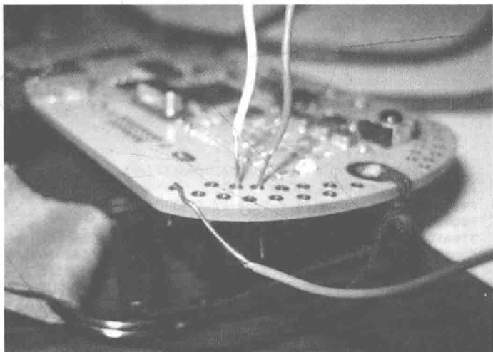
图7-25 DEFCON 20的Badge改装成的RS232-USB转接适配器
