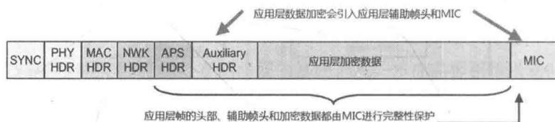
图6-10 使用了应用层安全机制的数据帧
