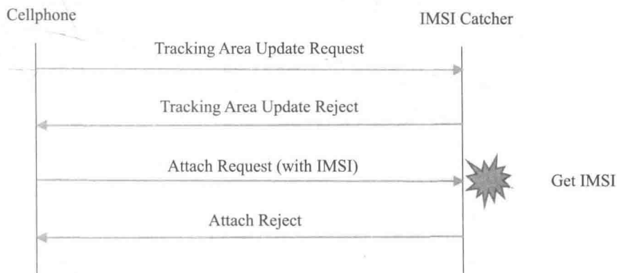
图7-13 信令大致流程图
