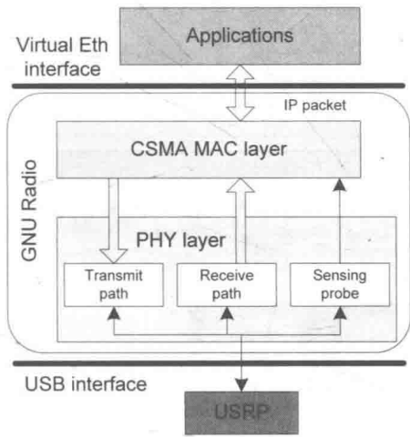
图9-21 Tunnel的系统框图
