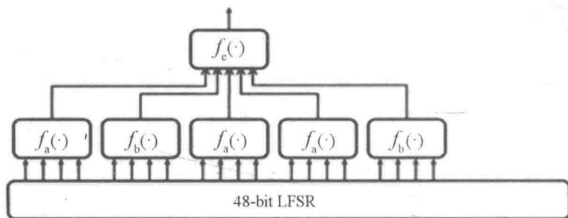
图2-4 过滤函数 f(x) 的构成
