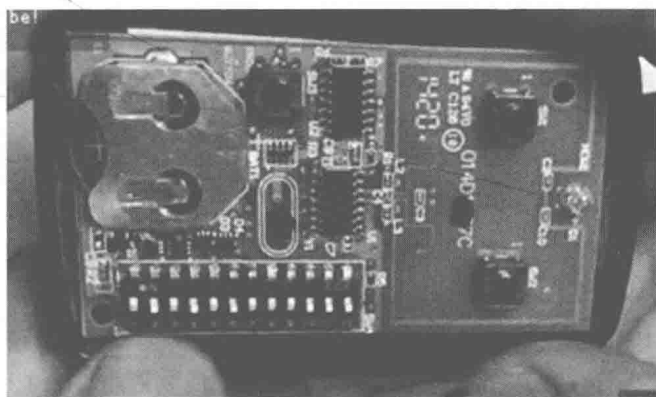
图3-9 遥控开关的内部结构
