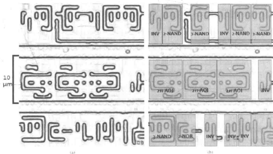
图2-2 “degate”脚本处理前后的电路照片对比
