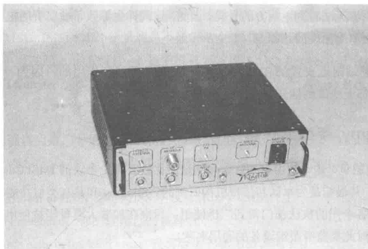
图7-15 便携式Stingray（又称KingFish）实物图
