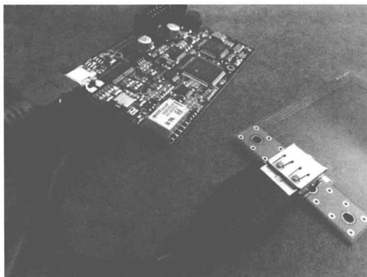
图2-16 连接天线至Proxmark III主板
