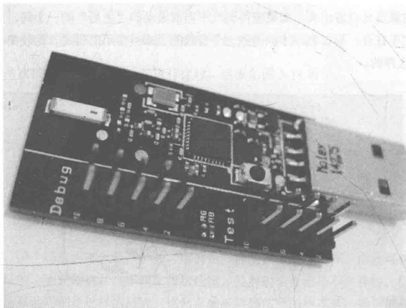
图3-21 播放工具RfCat
