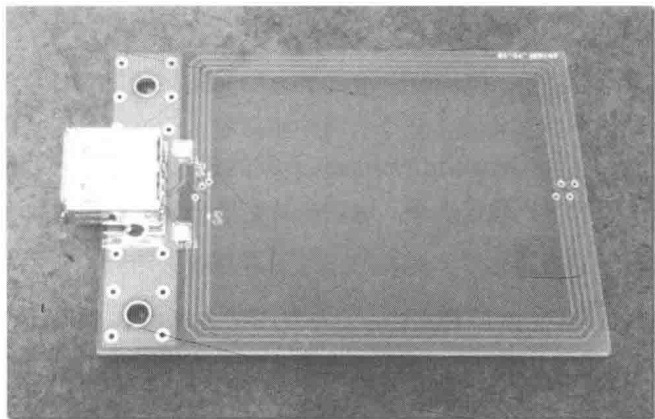
图2-6 与Proxmark III配套的高频读卡天线
