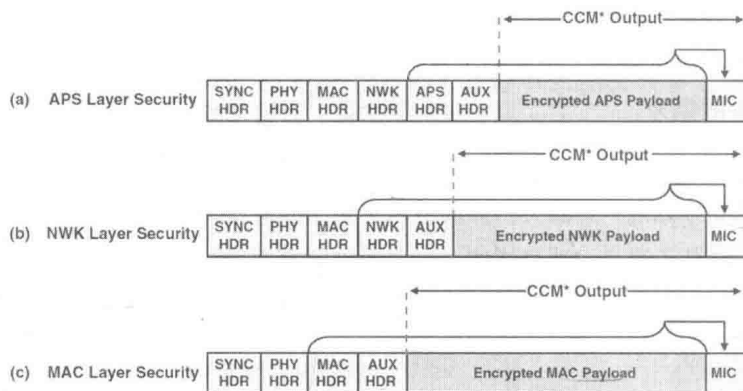
图6-8 ZigBee设备在三个逻辑层加入安全机制 6
