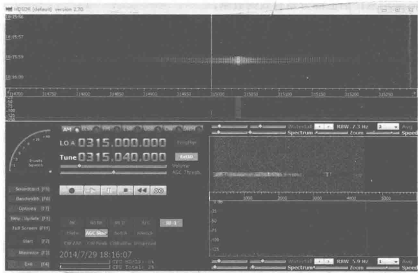
图3-13 某奥迪车钥匙信号频谱图
