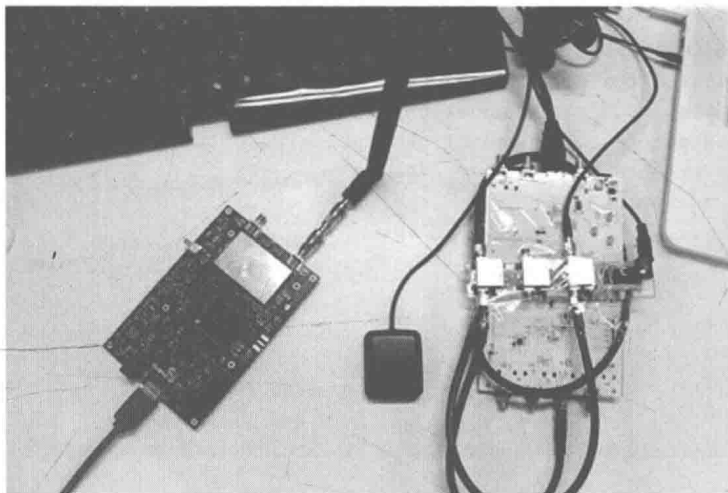
图8-14 回环测试
