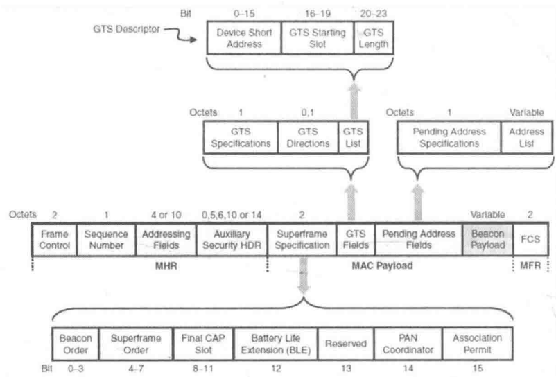
图6-24 信标帧结构
