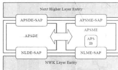
图6-6 应用支持子层的结构
