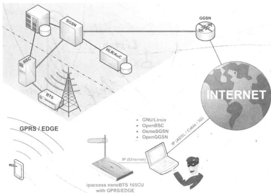
图7-3 GSM主动攻击结构图
