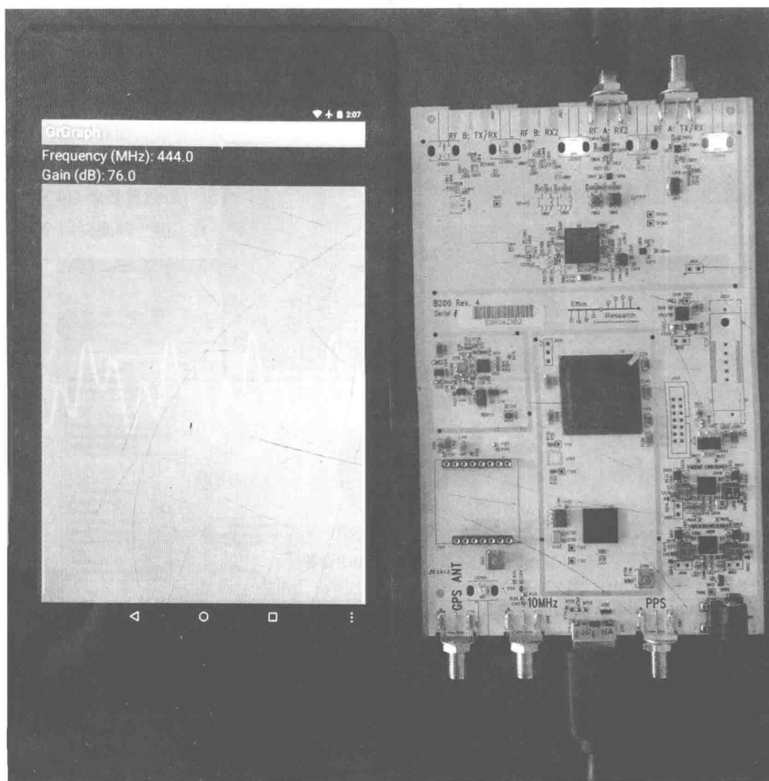
图9-8 Nexus 7 和一个USRP B200（不是mini版），运行GNU Radio安卓版本
