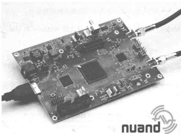
图9-11 bladeRF
