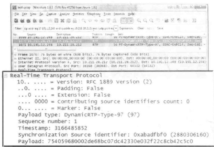
图7-26 UDP报文的Wireshark解析图（RTP协议）
