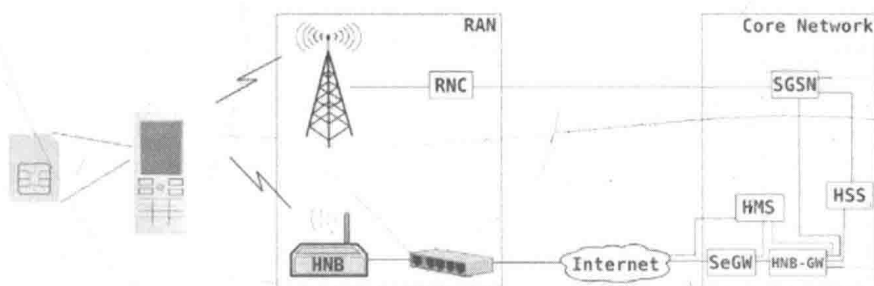
图7-51 家庭基站系统架构图
