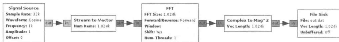
图9-17 FFT处理流图
