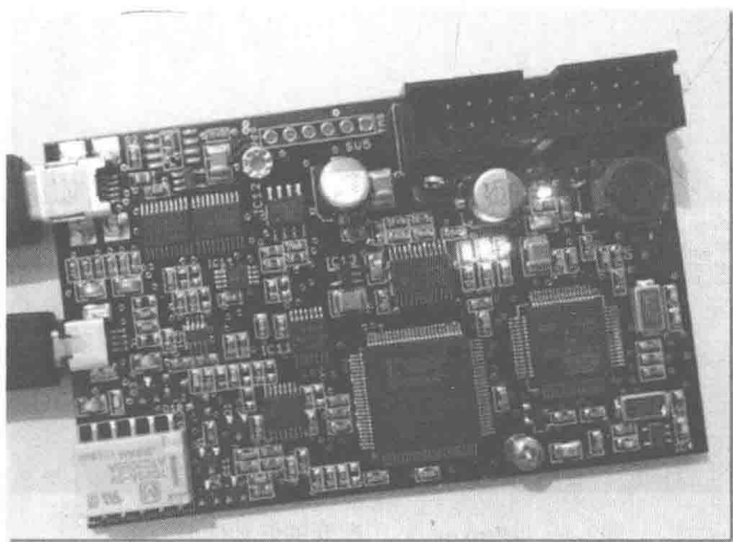
图2-5 Proxmark III裸板近照
