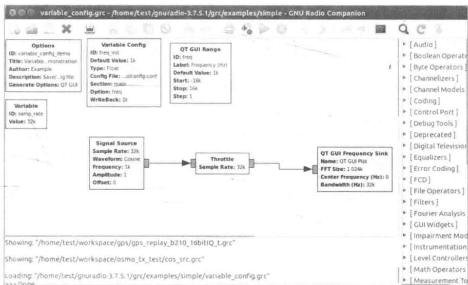
图9-14 variable_config.grc例子
