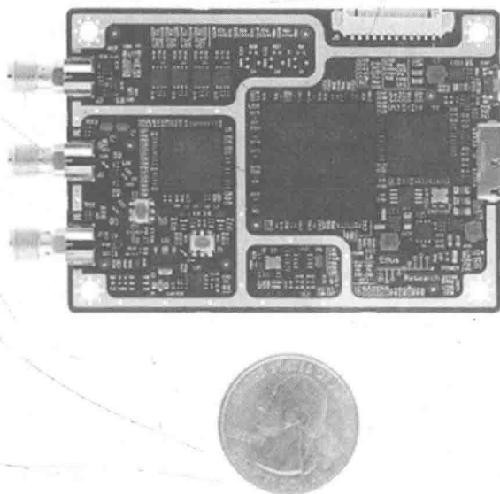
图9-7 B系列USRP设备
