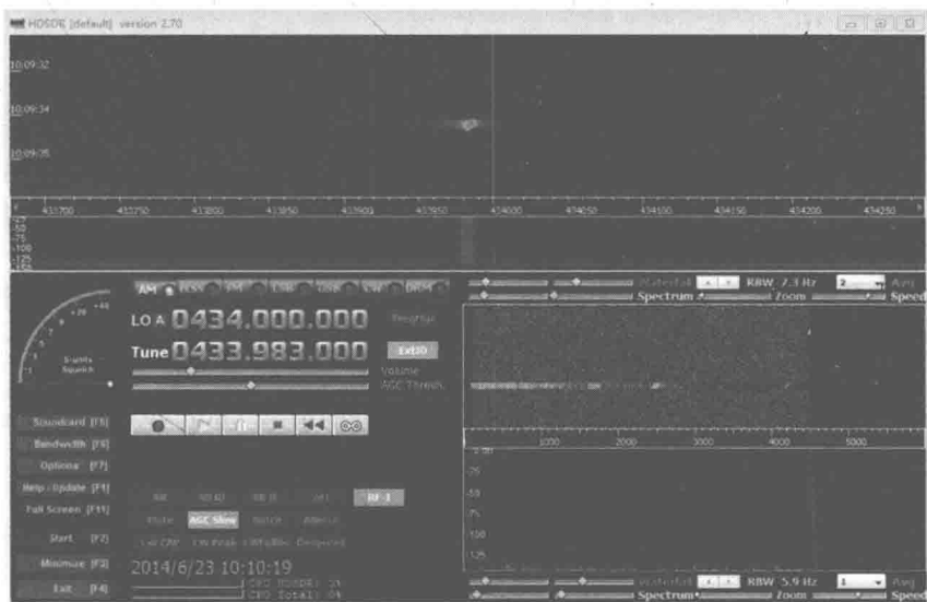
图3-5 遥控钥匙发射信号的频谱图
