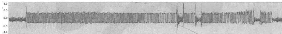
图3-29 胎压信号时序波形图
