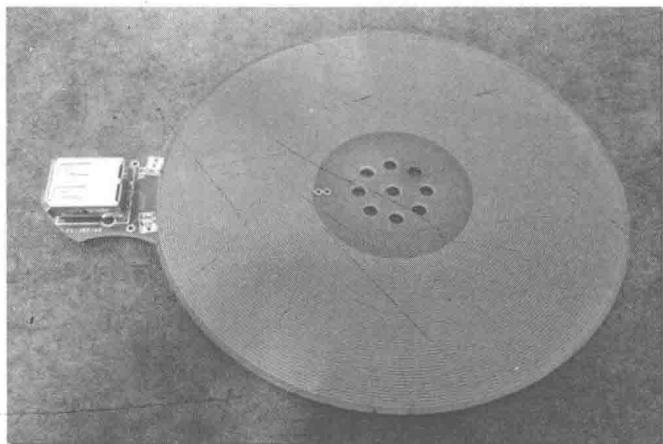
图2-7 与Proxmark III配套的低频读卡天线
