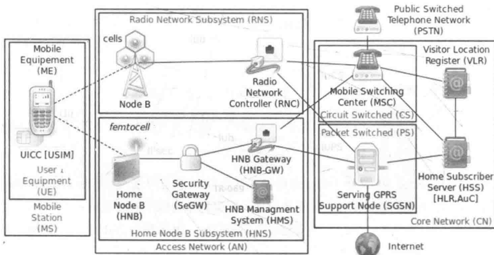
图7-21 家庭基站网络结构图
