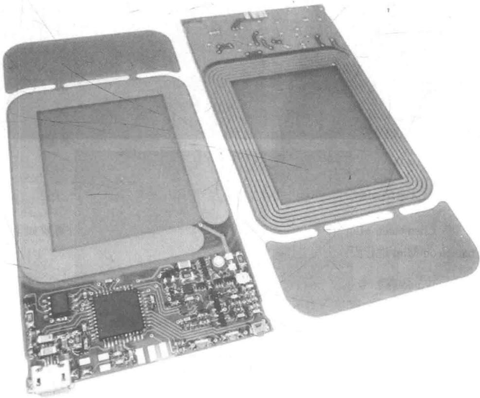
图2-28 Chameleon-Mini早期版本实物图
