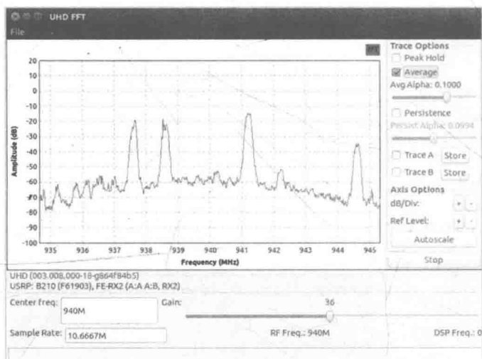
图9-13 使用 uhd_fft 观察 GSM 频段的信号频谱
