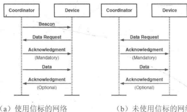
图6-45 ZigBee协调器向网络中其他节点发送数据的流程图 9
