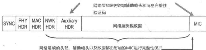
图6-9 使用了网络层安全机制的数据帧
