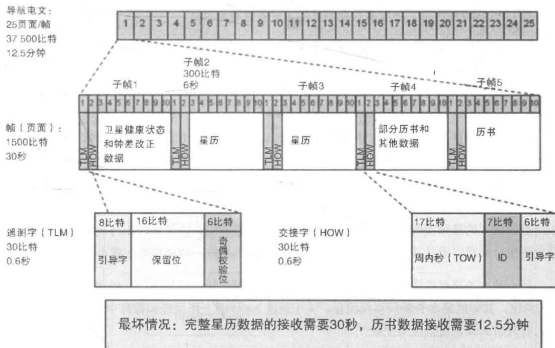
图8-10 GPS导航电文层次结构图
