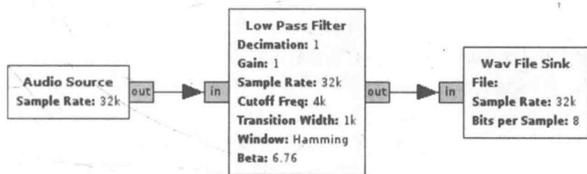
图9-16 音频处理流图
