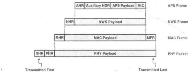
图6-2 ZigBee数据帧结构图 2
