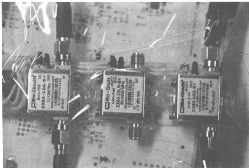
图8-12 带LNA和GPS Active天线的接收机
