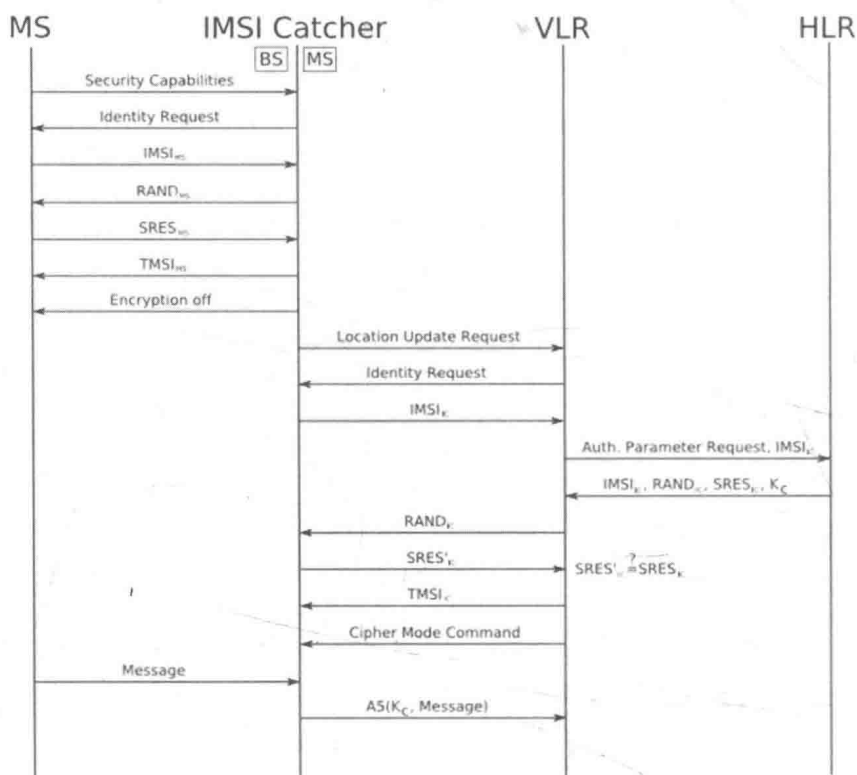
图7-9 GSM网络中的IMSI Catcher
