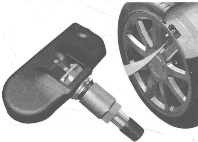
图3-27 胎压传感器
