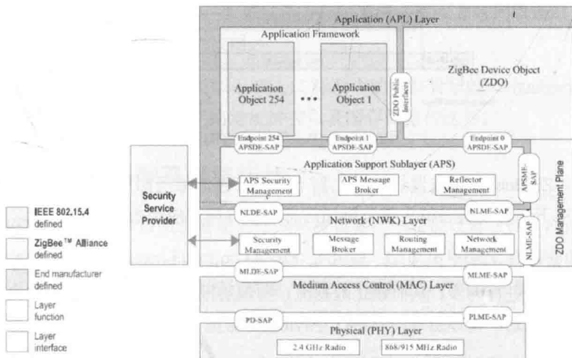
图6-1 ZigBee无线网络协议层次结构图 1
