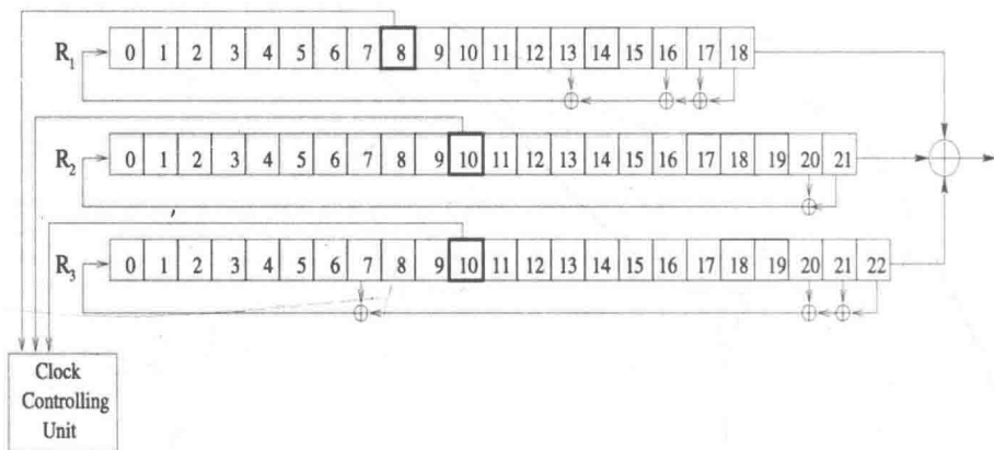
图7-2 A5/1算法结构示意图
