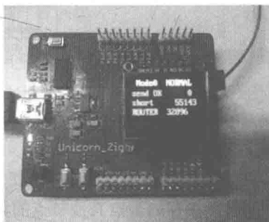
图6-43 ZigBee模块
