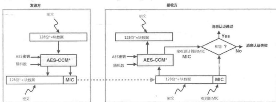
图6-7 在ZigBee中CCM*被用于数据加密及完整性认证
