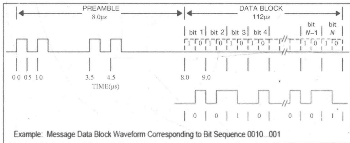
图4-1 前导脉冲部分
