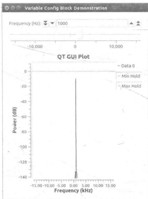
图9-15 余弦波形的频谱
