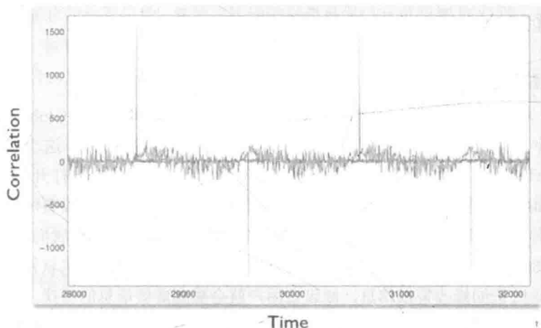
图8-32 解扩时原始信号与PN序列相关运算产生的相关峰
