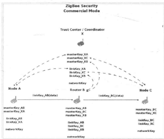
图6-11 高级安全/商用模式示意图
