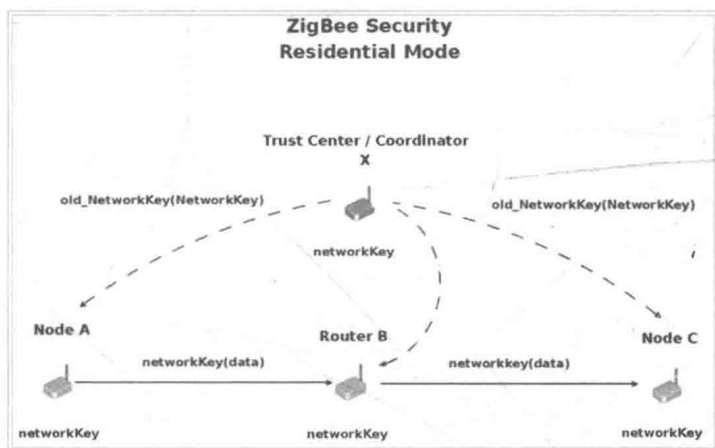
图6-33 ZigBee安全家用模式示意图
