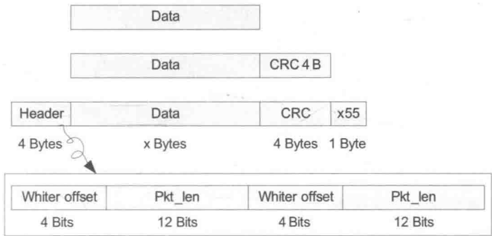
图9-22 IP数据包到MAC数据包的打包过程
