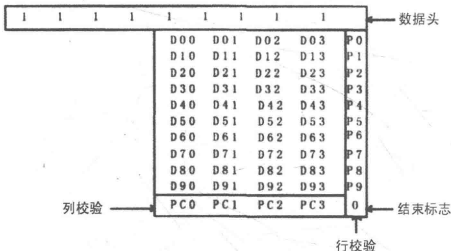
图2-38 ID卡64位数据结构
