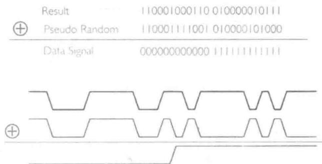
图 8-25 PN码解码过程
